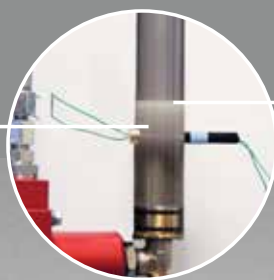
在实验室进行高压起 泡测试
