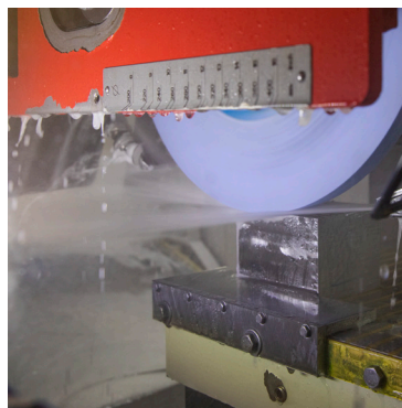
平面研削盤 (写真: Blohm 製)
