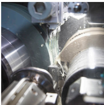
センターレス研削盤 (写真: Tschudin proLine 400)
