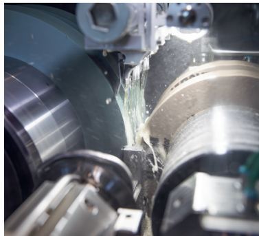
Rectificado sin centros (Imagen: rectificadora Tschudin proLine 400)
