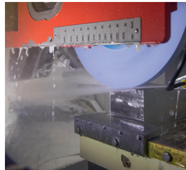
Rectificado de superficie (Imagen: rectificadora Blohm)
