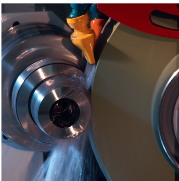
外圆磨削 (图为 Studer 机床)
