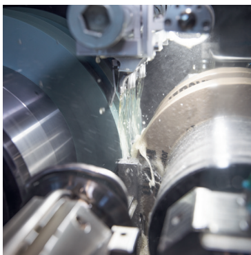
无心磨削 (图为 Tschudin proLine 400)
